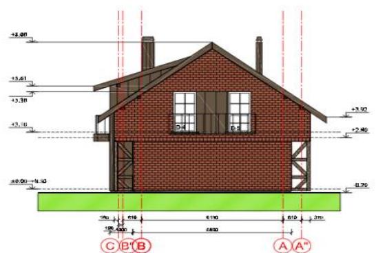
PASTATO FASADAS TARP AŠIŲ C-A", M1:100
